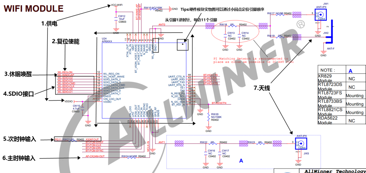
图 2-6: 模组引脚原理图
