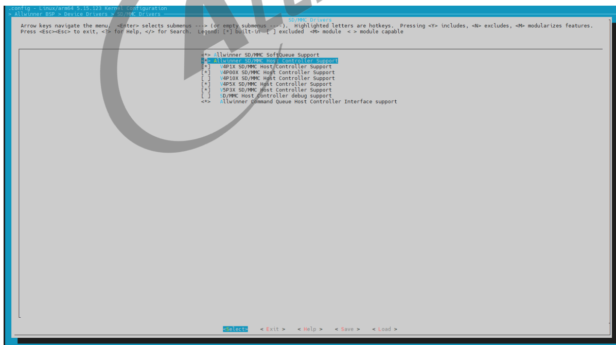
图 3-88: buildroot-sdc 配置
