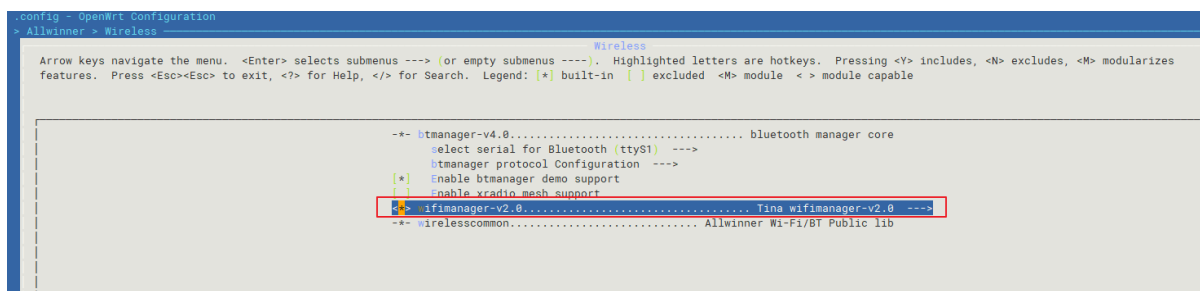
图 3-81: Tina5.0-wifimanager 配置
