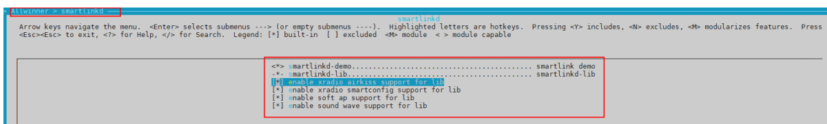
图 3-8: Tina-smartlinkd 配置
