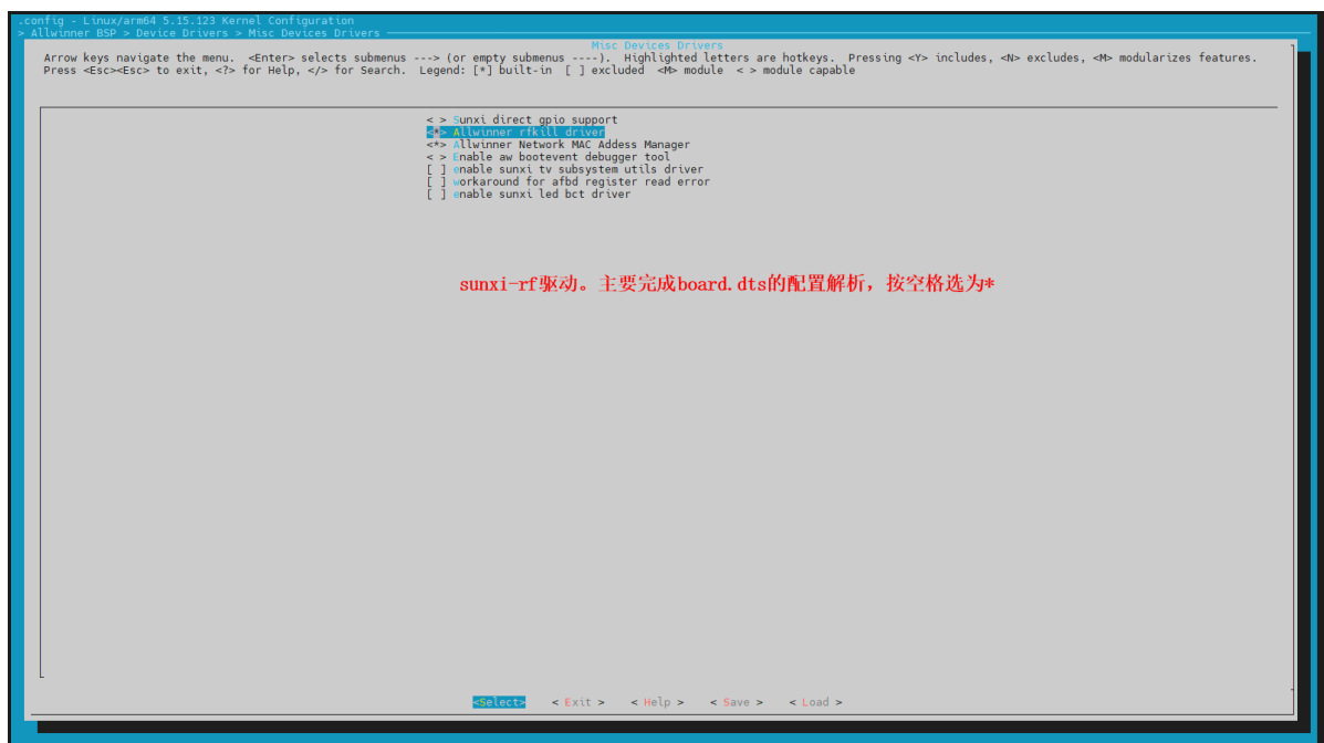
图 3-87: buildroot-sunxi-rf 配置
