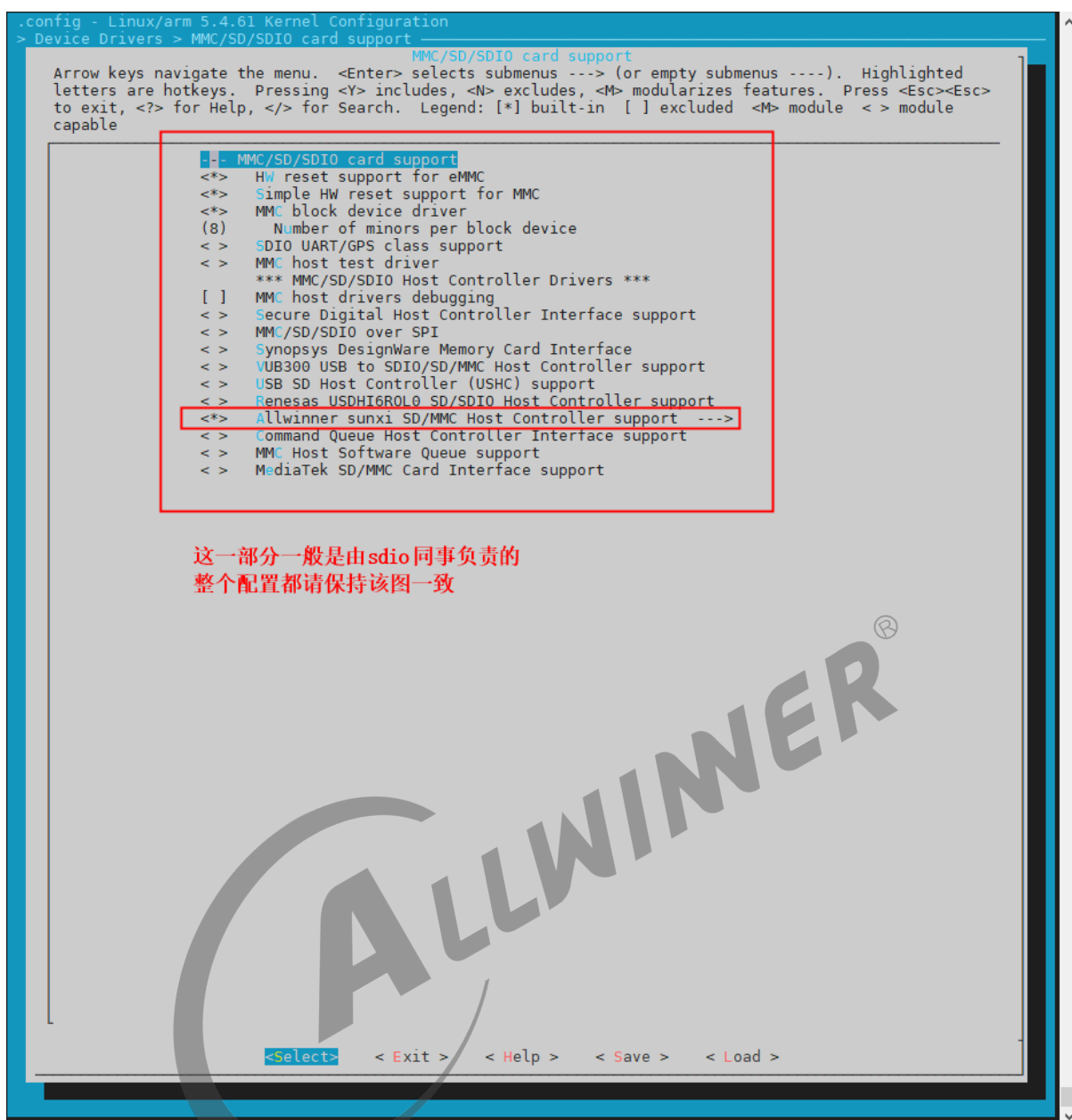
图 3-15: Tina-buildroot-sdc 配置
