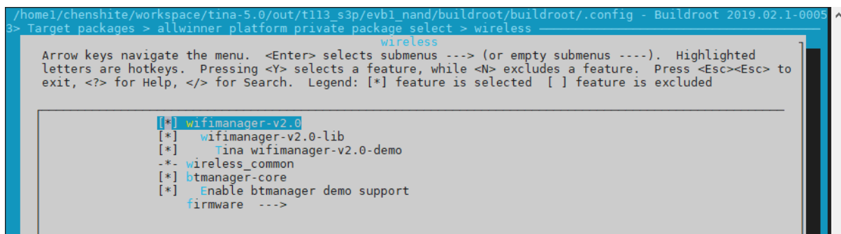
图 3-18: Tina-buildroot-wifimanager 配置
