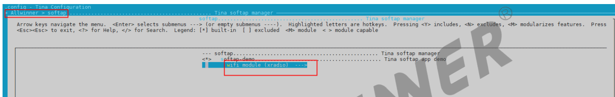
图 3-40: Tina-softap 配置
