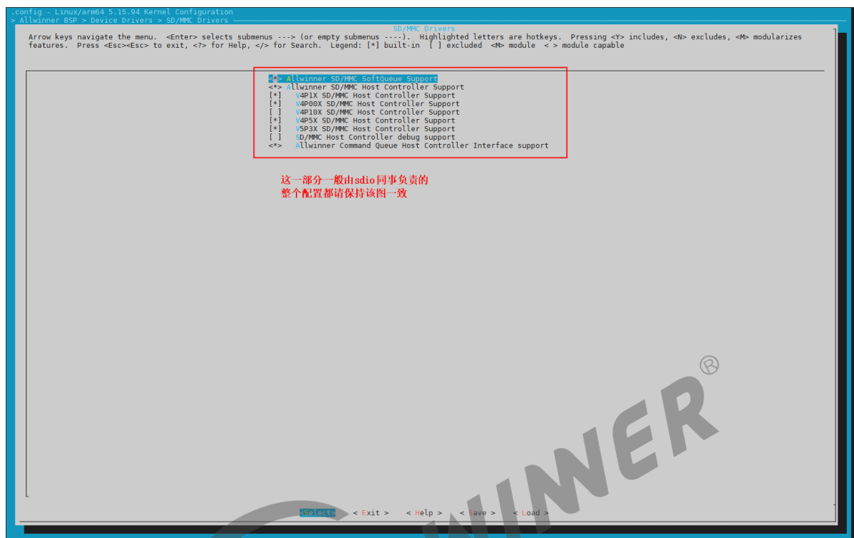
图 3-70: Tina-5.0-sdc 配置
