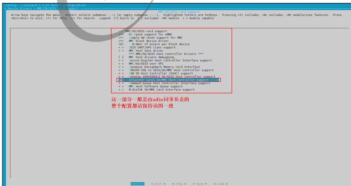
图 3-49: Tina-sdc 配置
