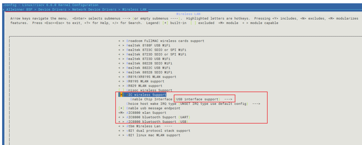
图 3-77: Tina5.0-aic_usb_sdio 内核配置
