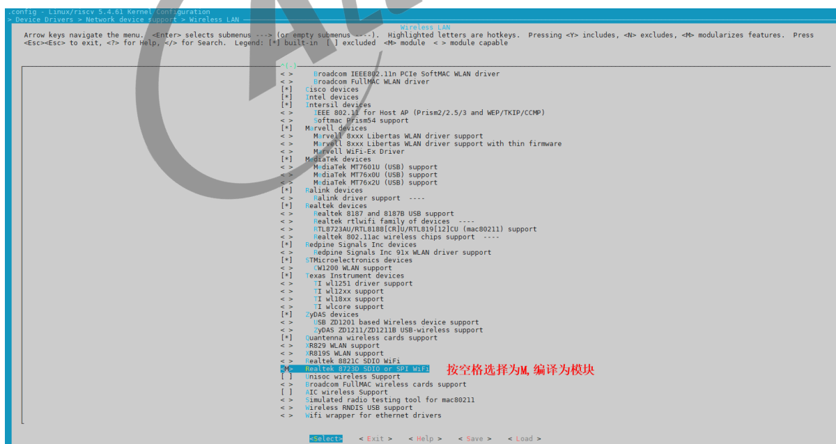
图 3-22: Tina-RTL8723DS 内核配置
