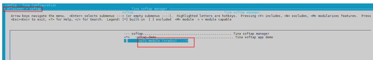
图 3-9: Tina-softap 配置
