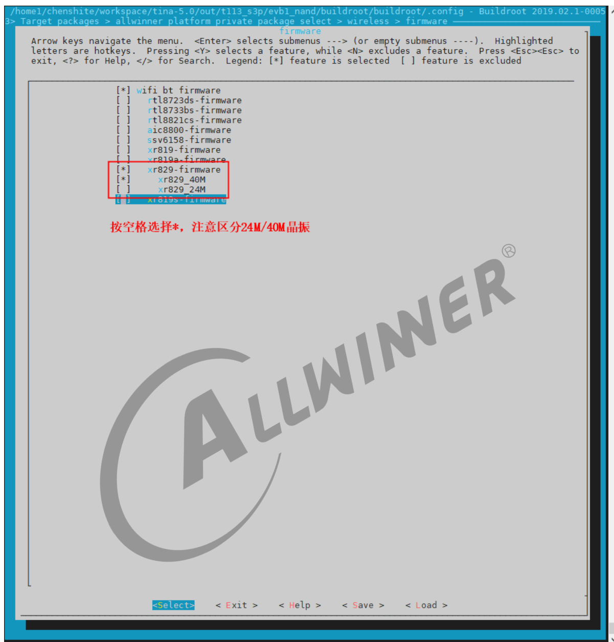
图 3-17: Tina-buildroot-XR829-firmware 配置
