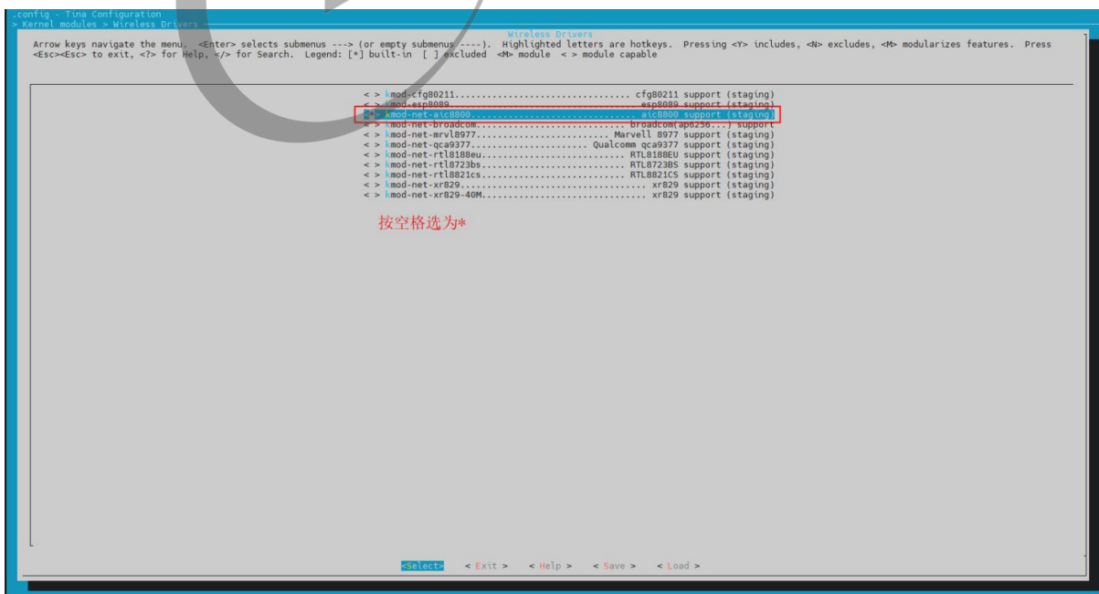
图 3-61: Tina-aic8800USB-module 配置
